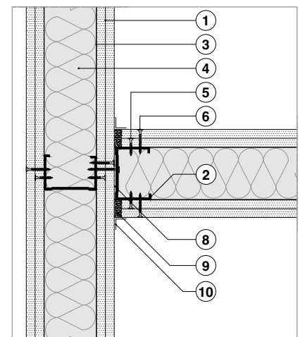
Rys. 21. Połączenie typu T – nie zalecane akustycznie
